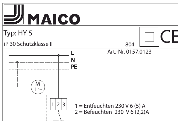
Verdrahtungsschema
