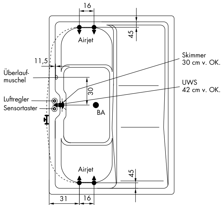
Standard-Positionen für Einbauteile
