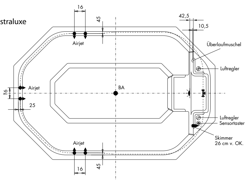
Standard-Positionen für Einbauteile
